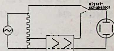
afb. 7, Vervorming versterker.
